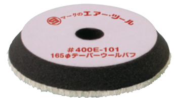
Φ165 ウールバフ 外径165×内径30×厚26mm
